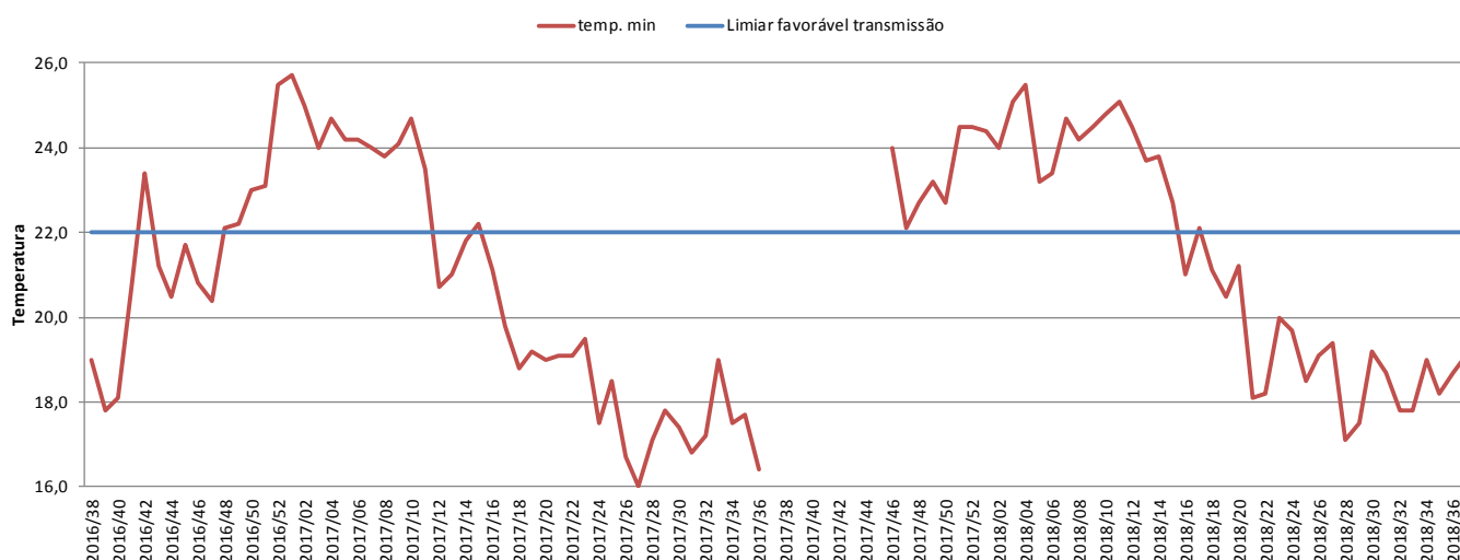
Gráfico 3 – Condições climáticas para transmissão das arboviroses
