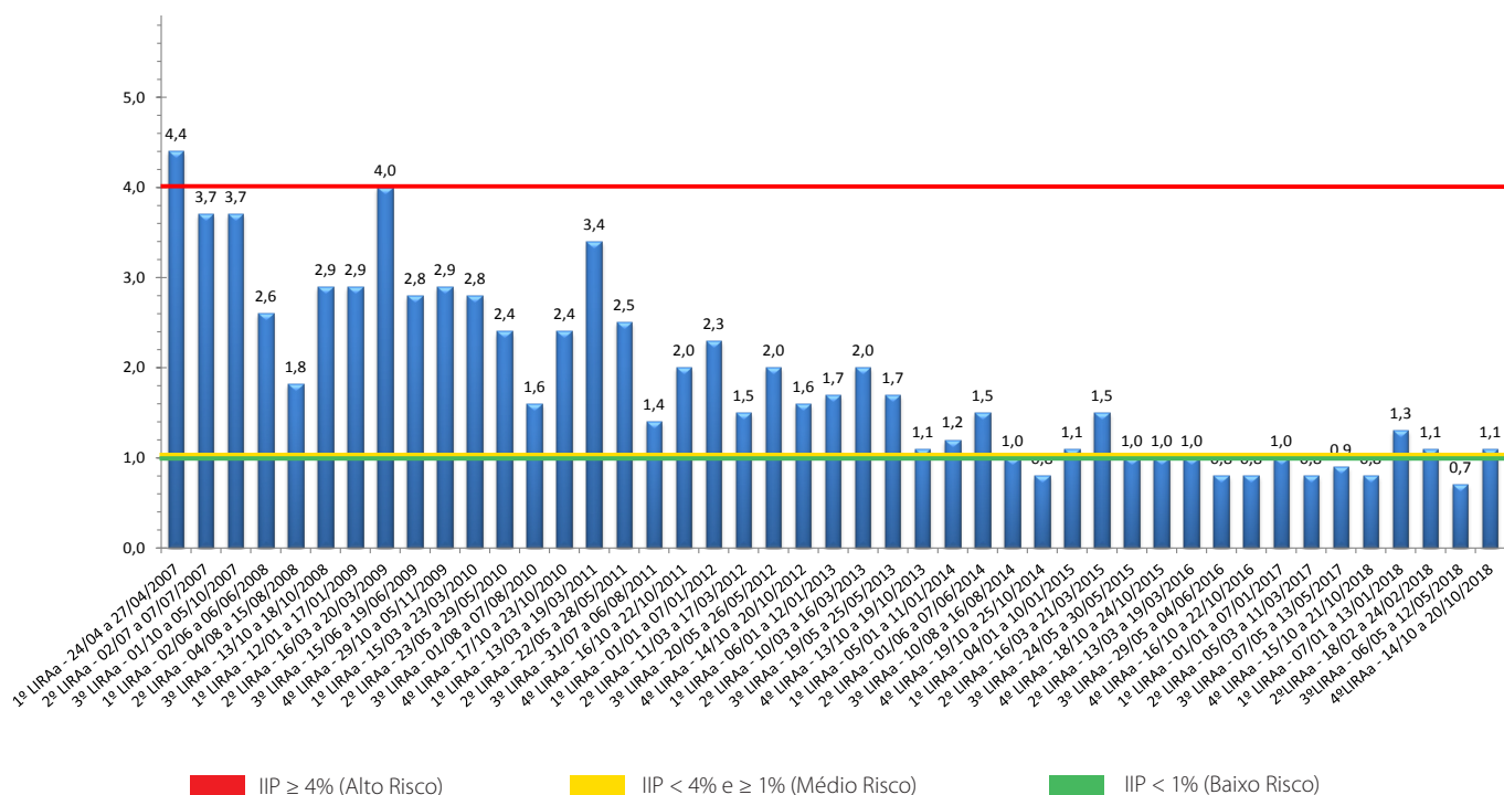
Gráfico 4 – Série histórica do Índice de Infestação Predial (%) do Município do Rio de Janeiro, 2007-2018
