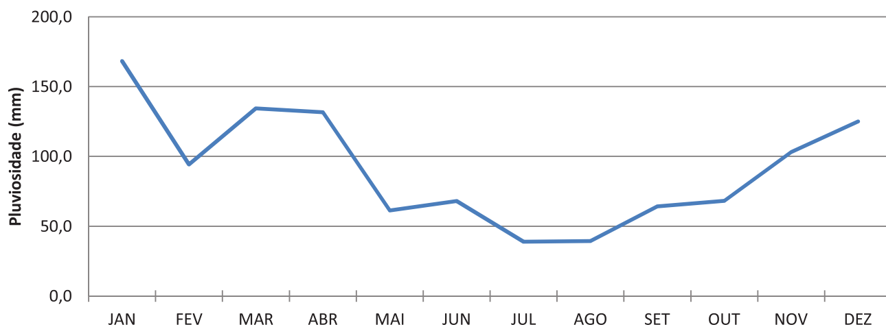
Gráfico 2 – Mediana da pluviosidade por mês, 2008-2017
