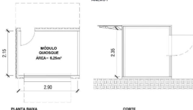
PLANTA BAIXA
