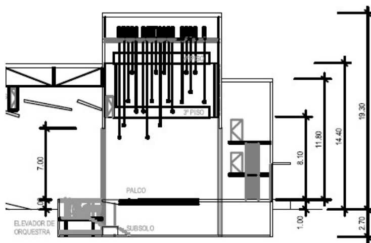
Fig. 3 – CORTE TRANSVERSAL - ÁREA CÊNICA
