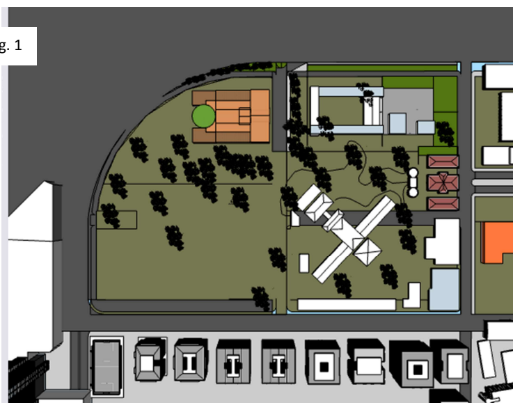
EQUIPAMENTO CULTURAL MULTIUSO – UFRJ - ESTUDO DE IMPLANTAÇÃO PROJEÇÃO ESTIMADA DO EDIFÍCIO – 65,00m X 46,00m
