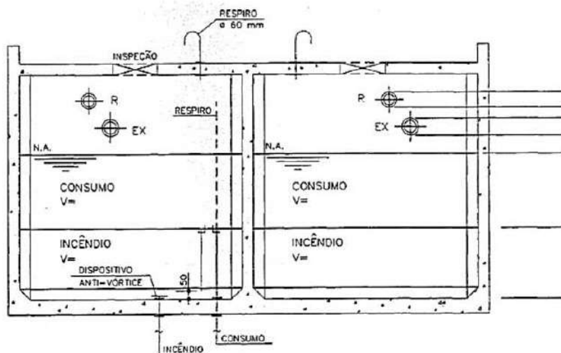
Detalhe esquemático do posicionamento das tubulações
