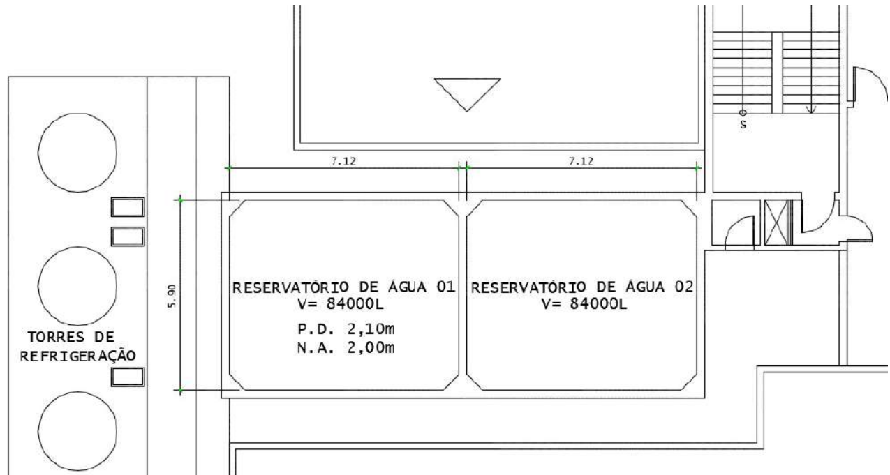
PLANTA BAIXA DOS RESERVATÓRIOS 01 E 02
