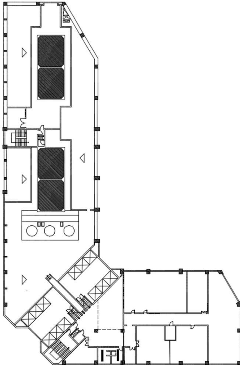
LOCALIZAÇÃO DOS RESERVATÓRIOS NO 12º PAVIMENTO
