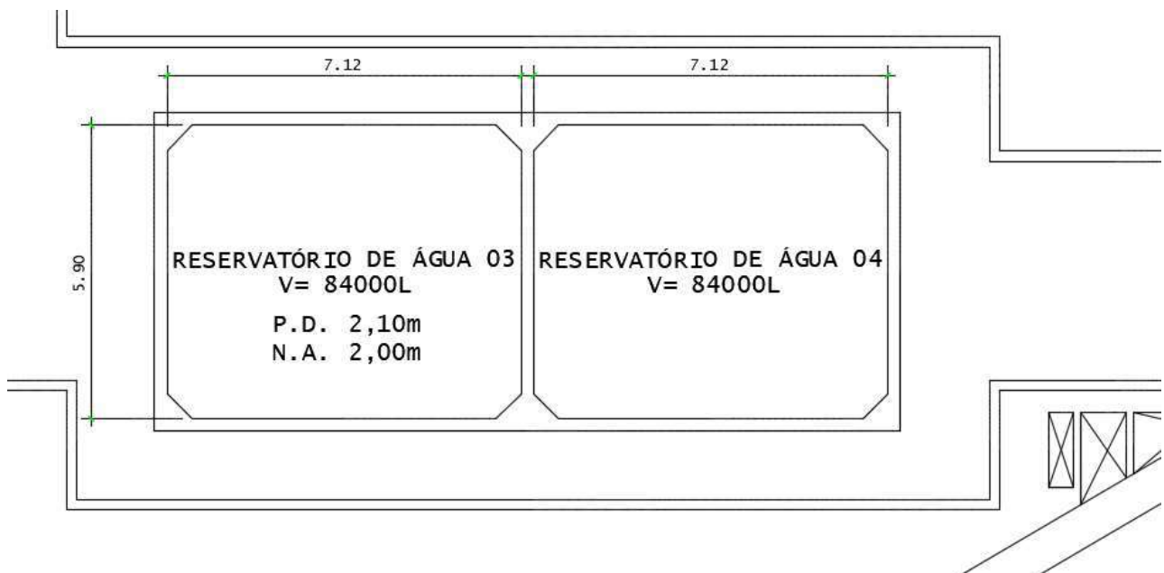
PLANTA BAIXA DOS RESERVATÓRIOS 03 E 04
