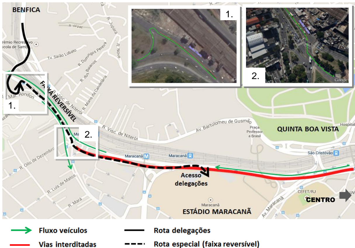
Figuras 12 e 13. Faixa reversível montada no dia do jogo da Final da Copa e detalhes
